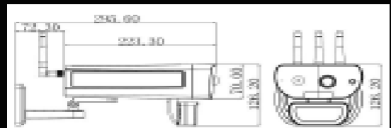
Tamaño:295.6MM*132MM*126.2MM
